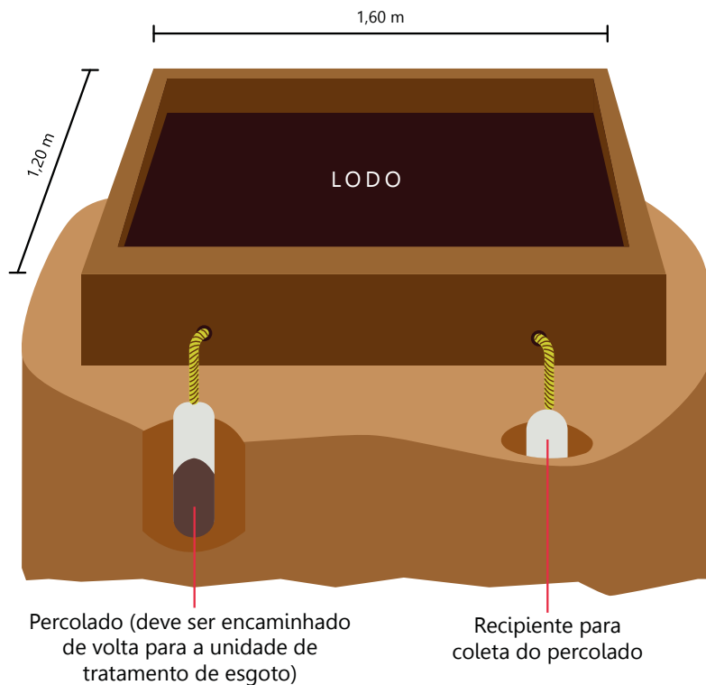
FIGURA 46. Leito de secagem de lodo simplificado proposto pela FUNASA (2014).
