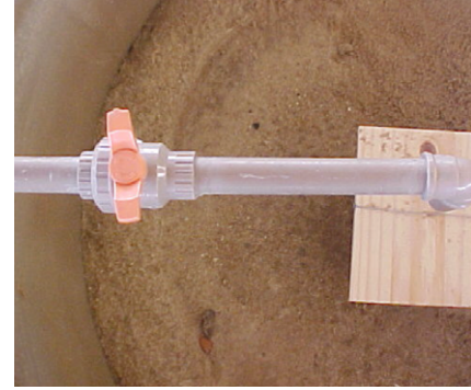
FIGURA 2. Filtro de areia construído em anéis de concreto para tratamento de esgoto vindo de um tanque séptico (Foto: Luana Cruz).
