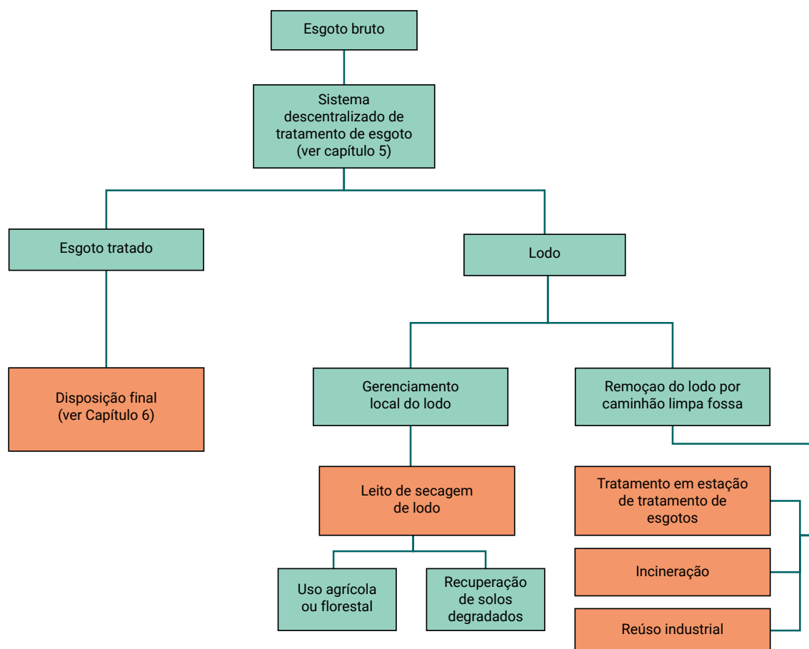
FIGURA 40. Alternativas para o gerenciamento do lodo gerado por sistemas descentralizados de tratamento de esgoto. Fonte: Elaborado pelos autores.
