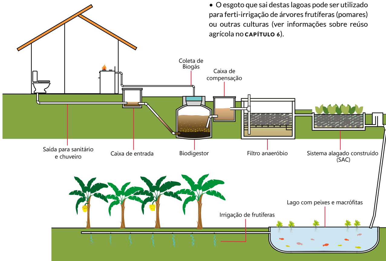
FIGURA 1. Esquema de biossistema integrado (BSI).
