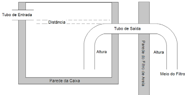
FIGURA 4. Esquema de caixa sifonada que gera aplicações do esgoto em pulsos no filtro de areia.
